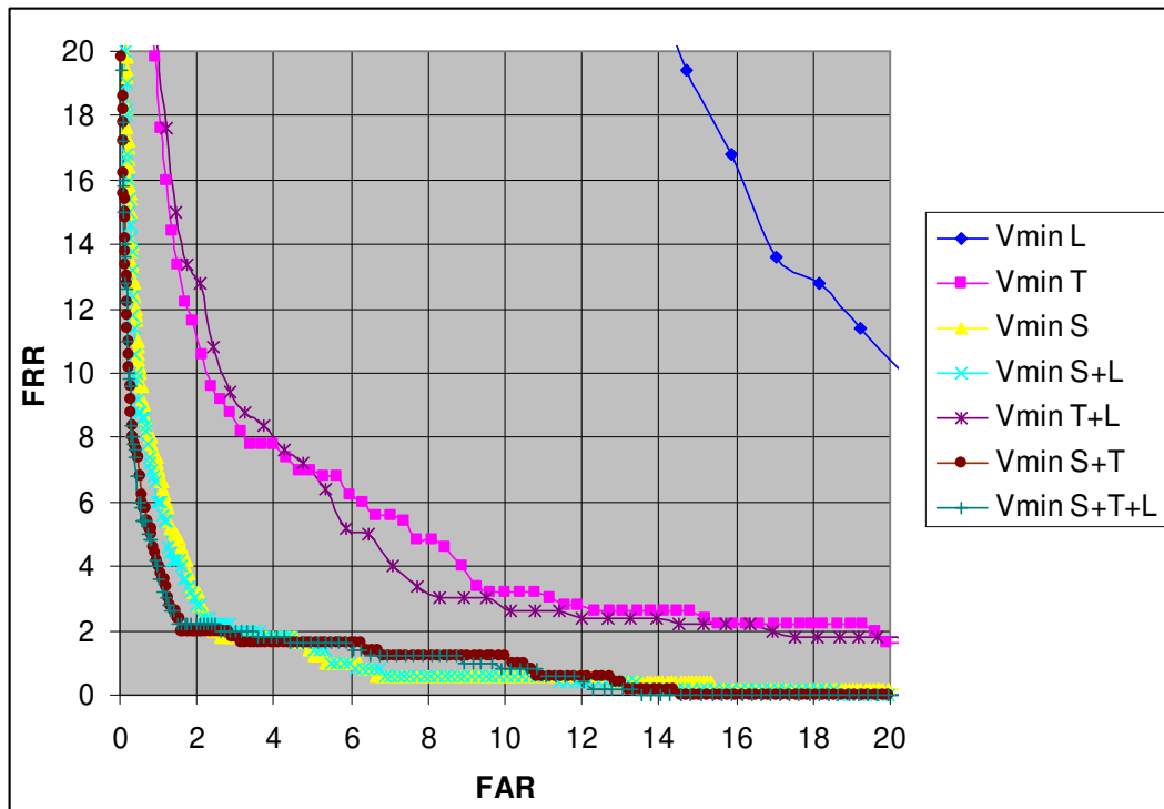
Figure 66. Comparatif des résultats obtenus sur la base ATOS (Palm) avec les différentes distances : spatiale (S), temporelle (T) et curviligne (L).
