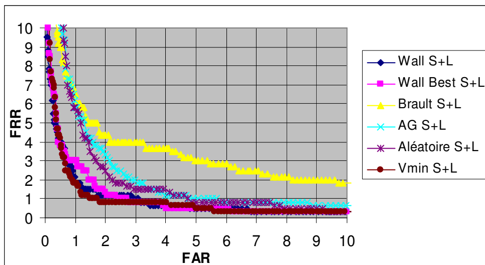
Figure 54. Résultats obtenus avec la combinaison des distances spatiale et curviligne pour chacune des méthodes présentées.
