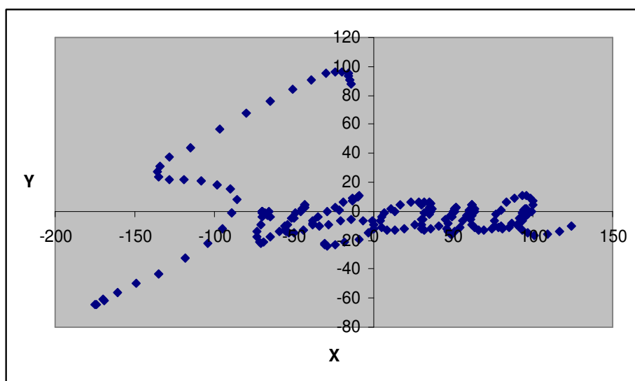
Figure 17. Translation pour positionner le centre de gravité à l'origine du repère.
