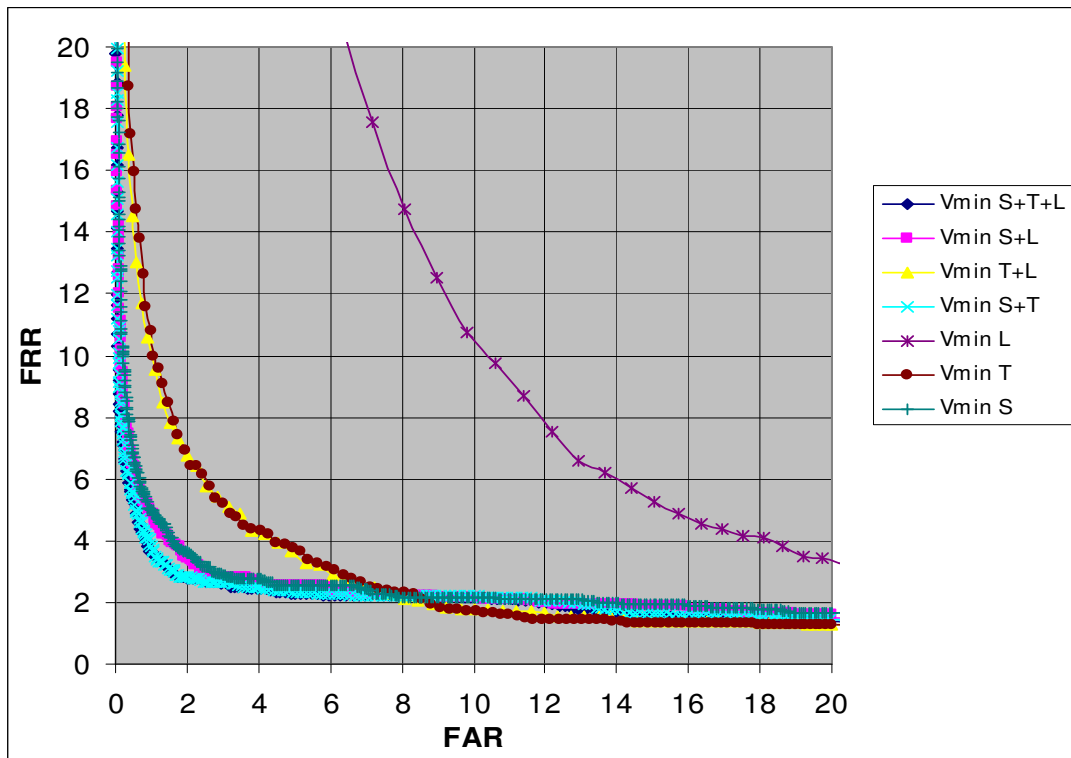
Figure 67. Comparatif des résultats obtenus sur la base MCYT avec les différentes distances : spatiale (S), temporelle (T) et curviligne (L).
