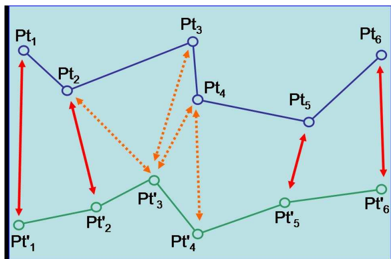
Figure 49. Illustrations des distances prises en considération : en rouge, les distances comptabilisées dans le calcul de la dissimilarité entre les signatures.
