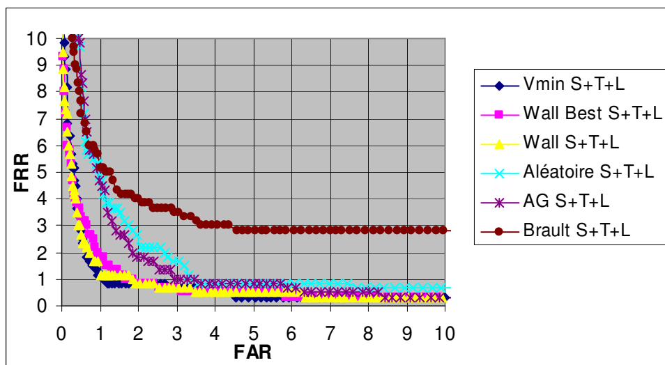
Figure 56. Résultats obtenus avec la combinaison des distances spatiale, temporelle et curviligne pour chacune des méthodes présentées.
