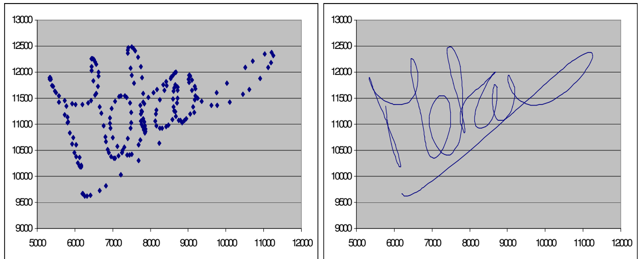
Figure 34. Signature avant et après Bresenham.
