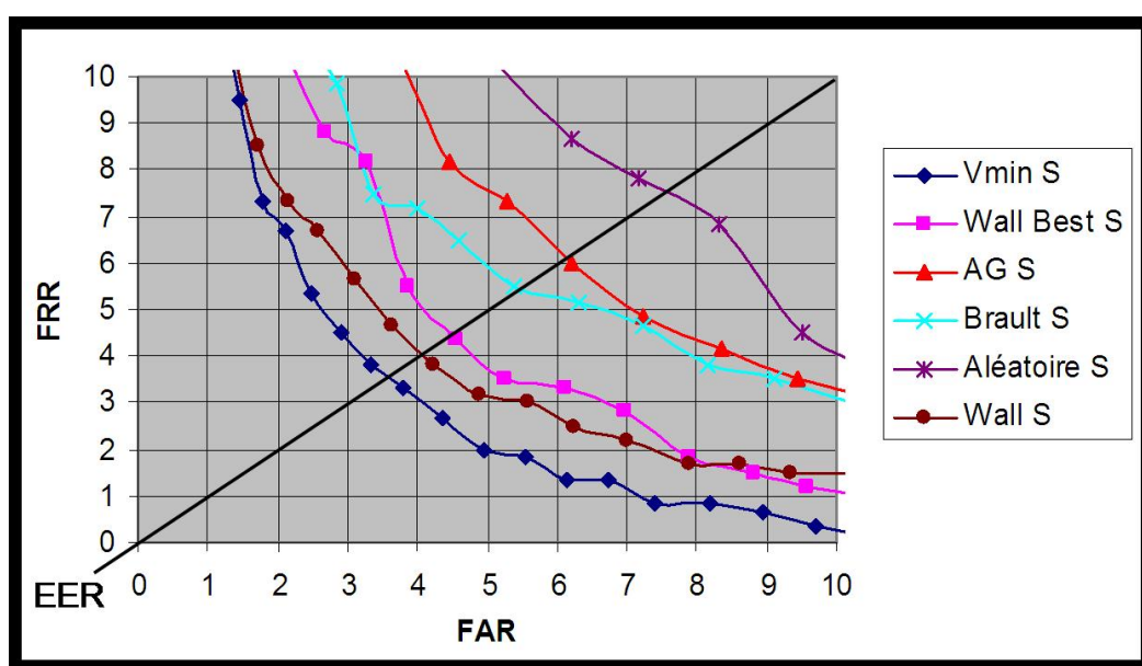
Figure 31. Résultats obtenus à partir de chacune des méthodes présentées (S=Spatiale) basées sur la distance calculée avec DTW.
