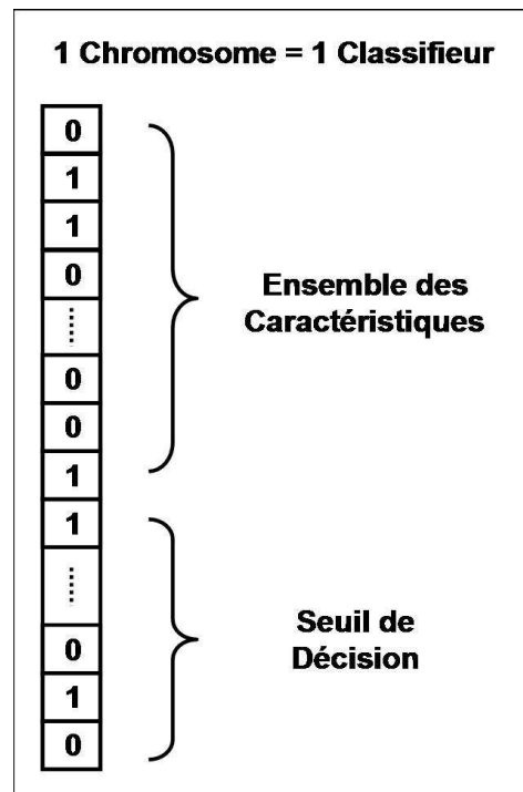
Figure 43. Illustration de la structure d'un chromosome i.e. un classifieur.
