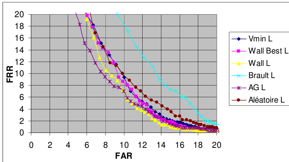
Figure 52. Résultats obtenus avec la distance curviligne pour chacune des méthodes présentées (L=Curviligne).
