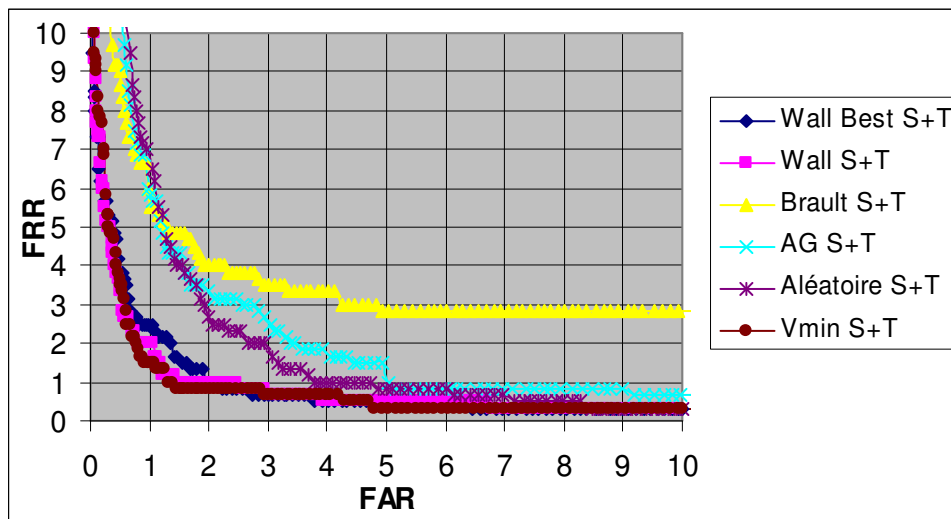
Figure 53. Résultats obtenus avec la combinaison des distances spatiale et temporelle pour chacune des méthodes présentées.
