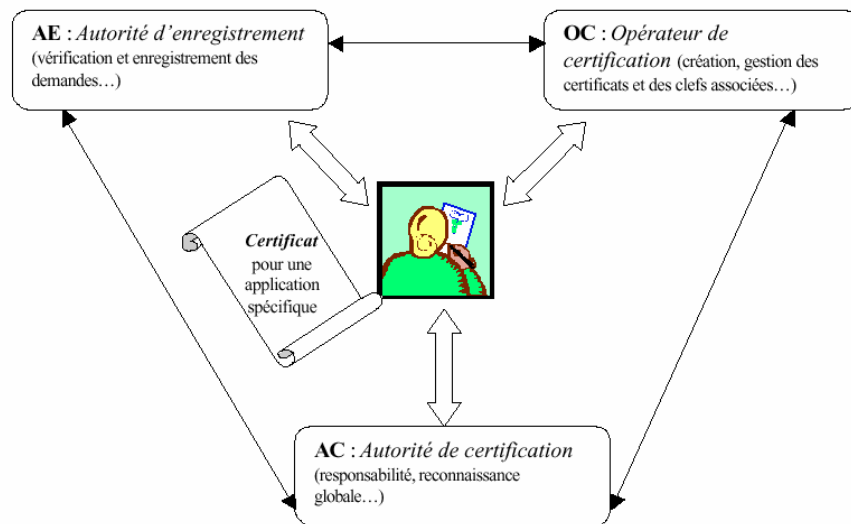
Figure 57. Architecture d'une Infrastructure de Gestion de Clés.
