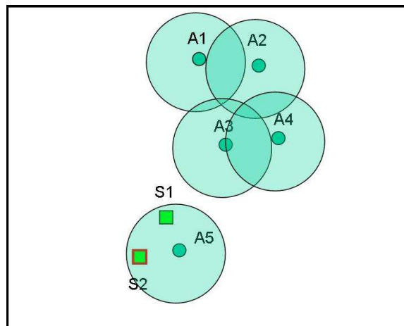
Figure 33. Modèle constitué de chacune des signatures d'apprentissage (● : signatures d'apprentissage, ■ : signatures à tester).
