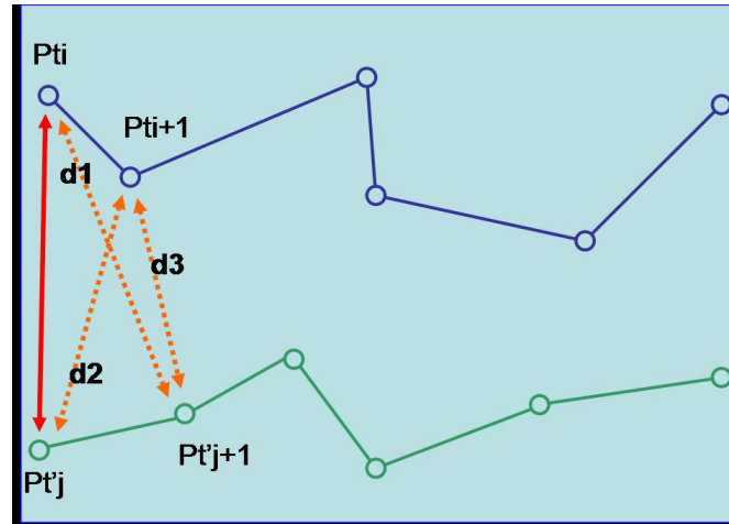
Figure 11. Principe de l'algorithme DTW.
