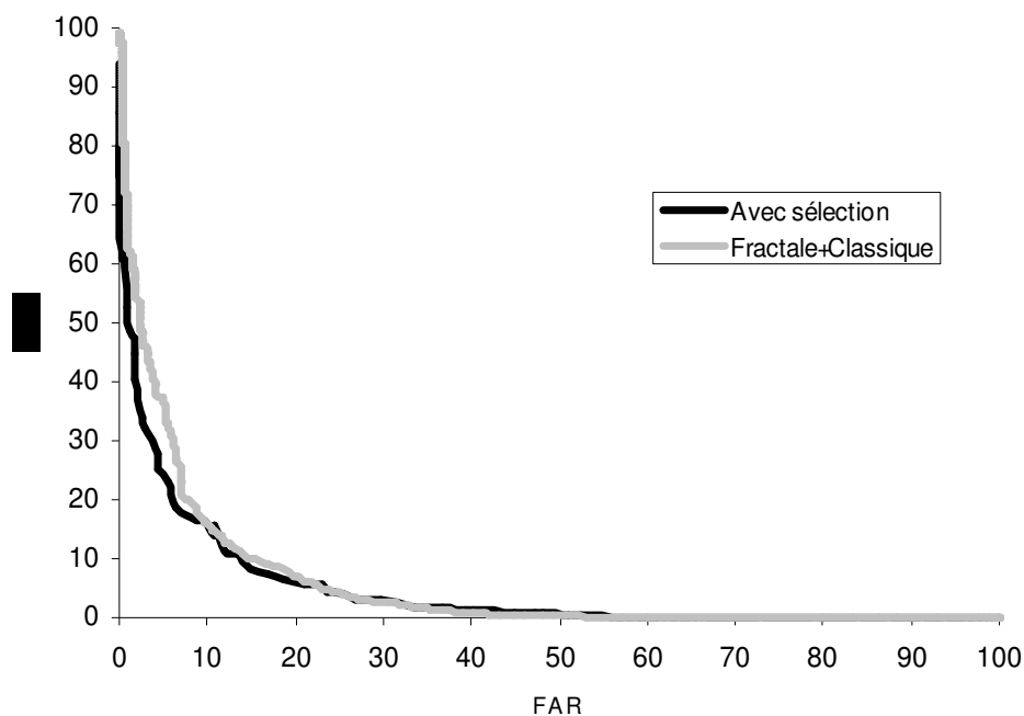
Figure 45. Comparaison des performances obtenues avec et sans sélection des caractéristiques par algorithme génétique multiobjectifs.
