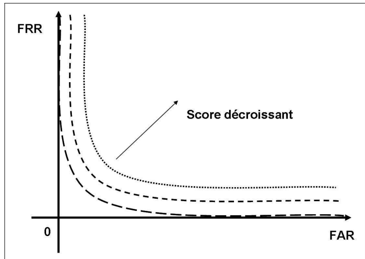
Figure 44. Illustration des courbes obtenues à partir de l'ensemble des chromosomes issus de la population.
