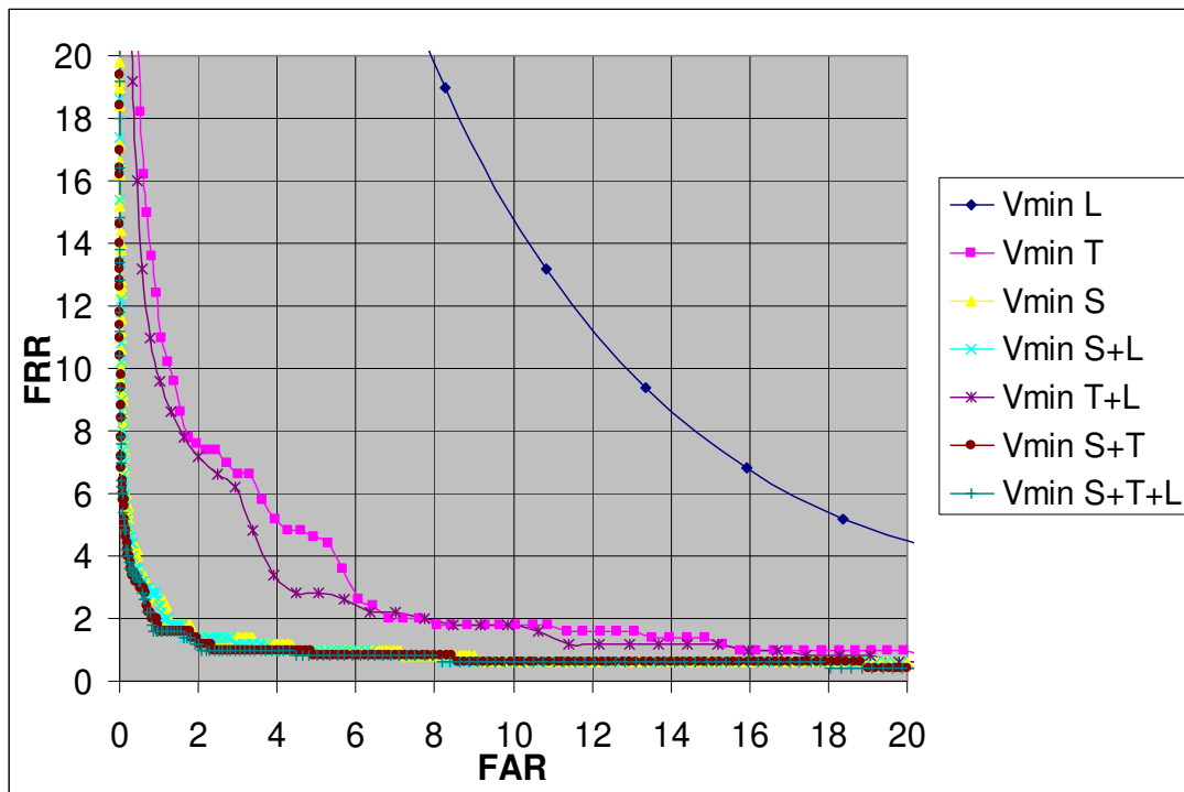
Figure 65. Comparatif des résultats obtenus sur la base ATOS (Tablet) avec les différentes distances : spatiale (S), temporelle (T) et curviligne (L).
