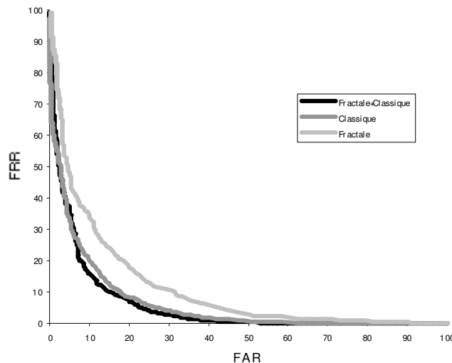
Figure 42. FAR vs FRR pour différentes valeurs de \alpha dans un système de vérification basé sur une représentation vectorielle des signatures.
