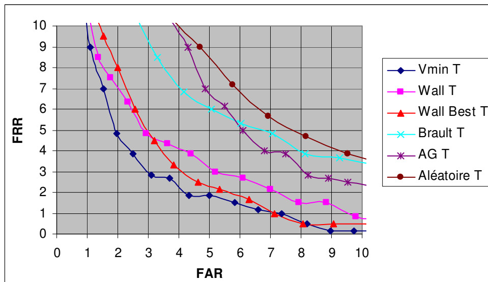
Figure 51. Résultats obtenus avec la distance temporelle pour chacune des méthodes présentées (T=Temporelle).
