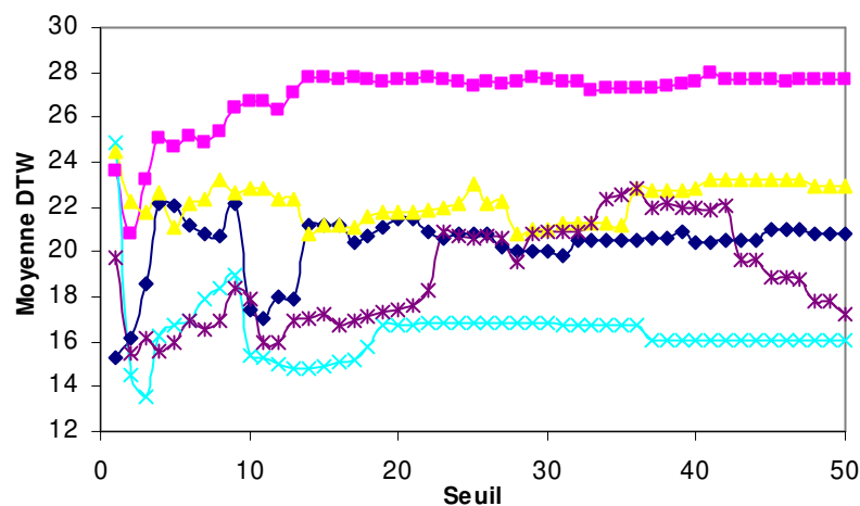
Figure 29. Illustration de l'évolution de la moyenne des distances DTW pour 5 signataires.
