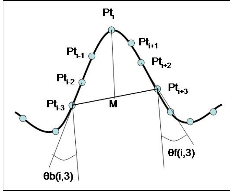
Figure 24. Illustration du calcul de la représentativité du point Pt_i avec n=3 .
