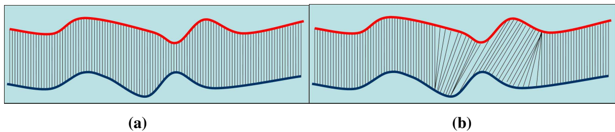
Figure 10. Mise en correspondance point à point entre deux signatures sans prise en compte des décalages temporels (a) et en appliquant l'algorithme DTW (b).
