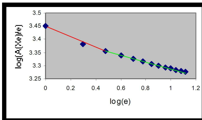
Figure 36. Evolution de l'aire des dilatés de la signature en fonction de la taille de l'élément structurant avec des échelles logarithmiques.
