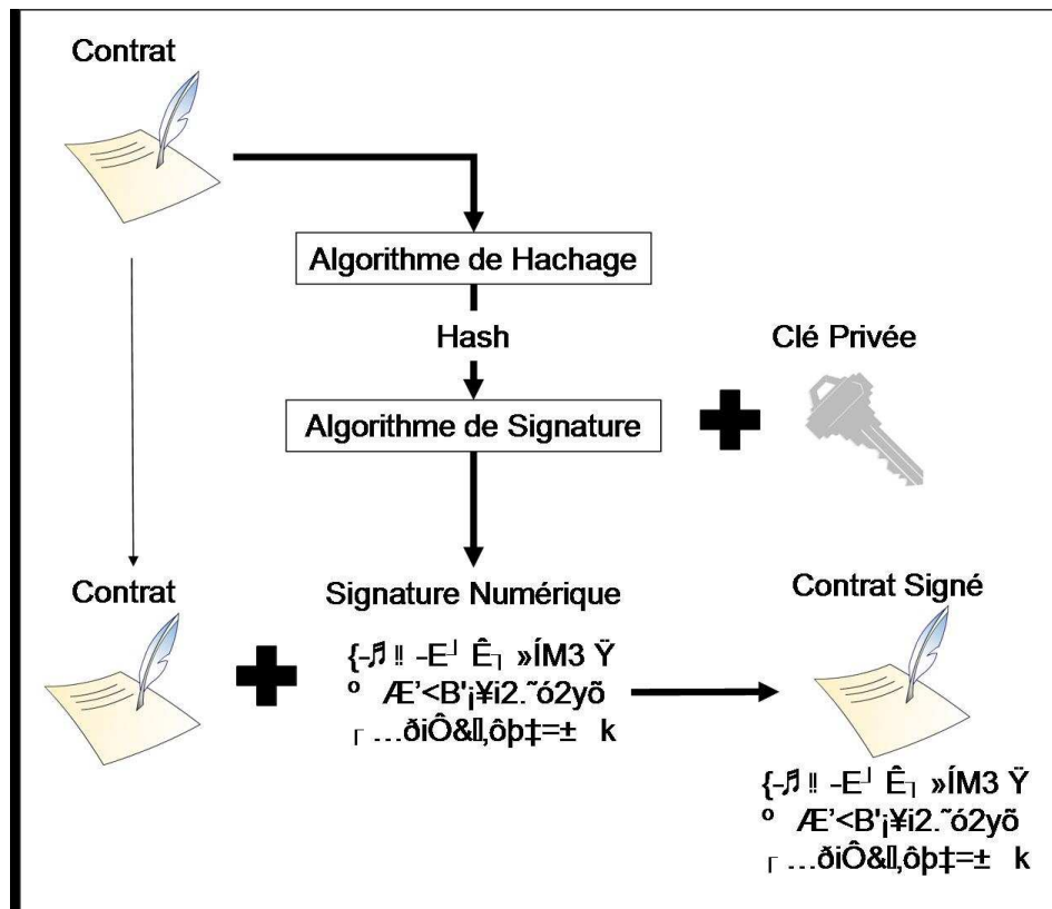
Figure 70. Etapes menant à la signature numérique d'un contrat.
